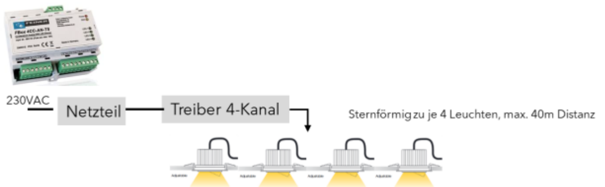
Beispiel: 4-Kanal LED-Treiber/Dimmer mit sternförmiger Verkabelung
