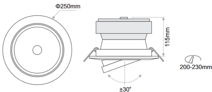
Leuchten-Beispiel ELECTRON RONELO für 200mm-230mm Deckenausschnitt und 250mm Leuchten-Außendurchmesser
